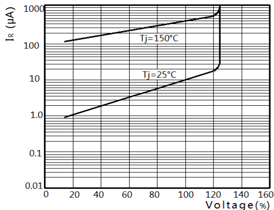
图 3. 典型反向特性
