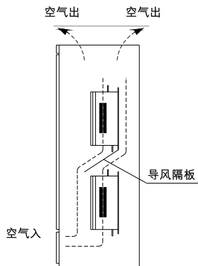
图3-3 纵向布局
