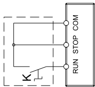
二线控制自由停车
