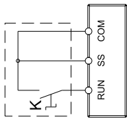
二线控制软停车
