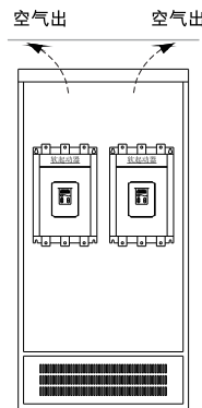
图3-2 横向布局
