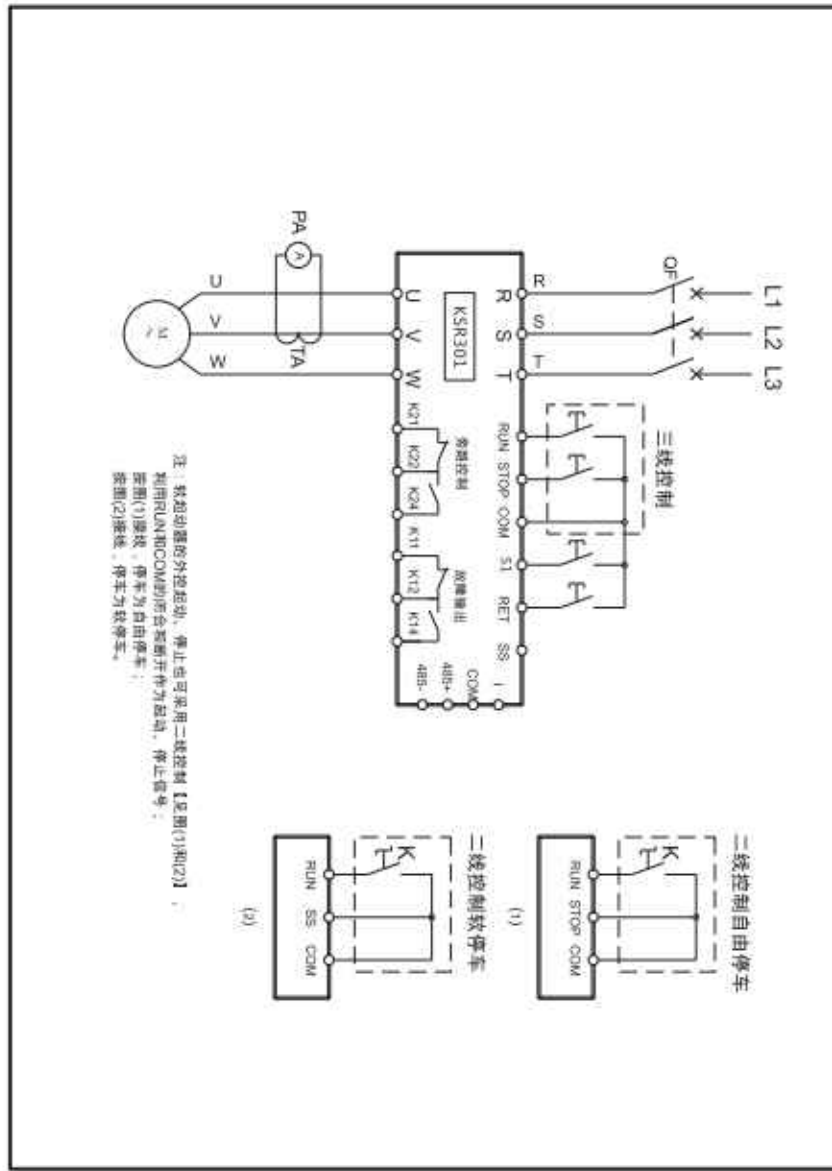
附录七：KSR系列301型软起动器典型应用接线图
