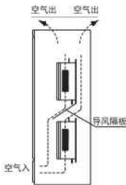
图3-3 纵向布局安装
