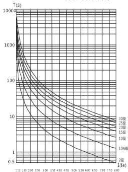
IEC60974-4-2电机热态保护曲线
