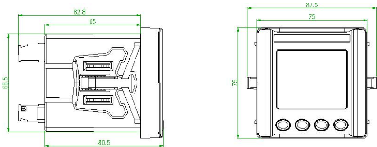
图 2 APM510 尺寸图
