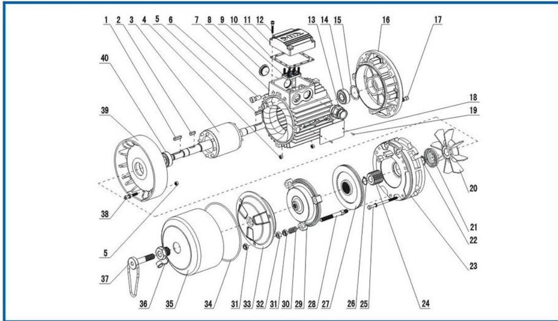
BMA部件分解图
