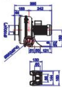
HTB75-032 2-stage
