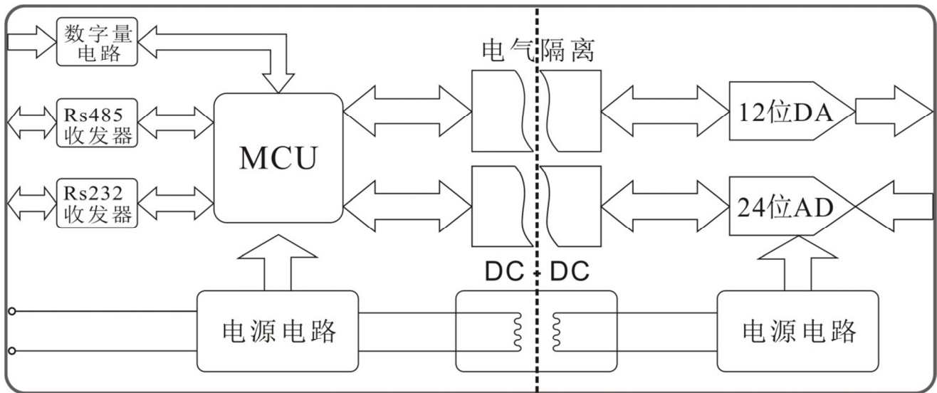
图 1-2 DAM-422X 工作原理框图
