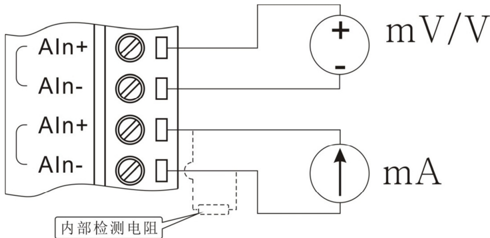
图 4-1 DAM-422X 模拟量输入接线示意图
