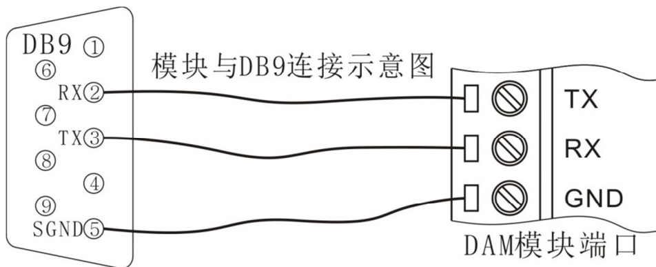
图 7-1 DAM 模块与 PC 机连接示意图
