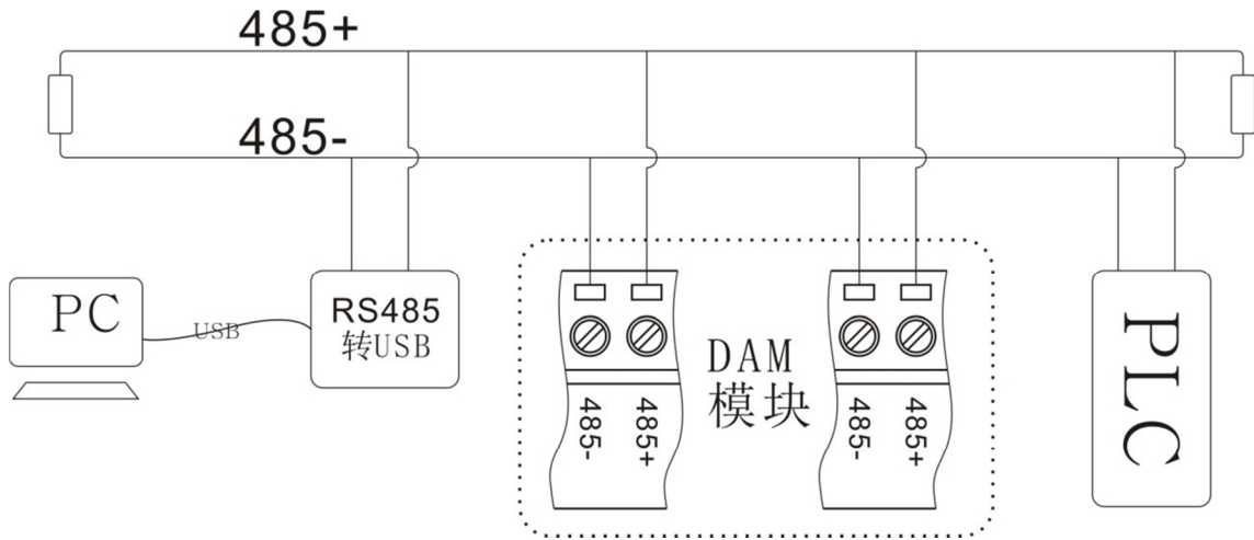
图 7-2 DAM 模块通过 RS485 接口与其它设备组网连接示意图
