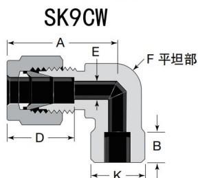
卡套90° 承插焊直角
