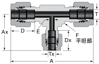
卡套变径三通 SKTB
