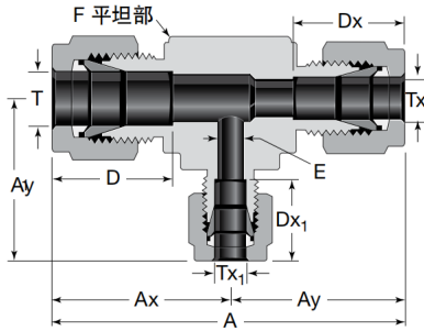
卡套变径三通 SKTB
