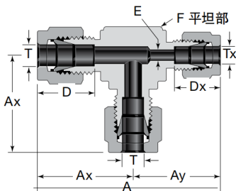
卡套变径三通 SKTB
