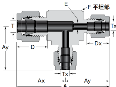
卡套变径三通 SKTB
