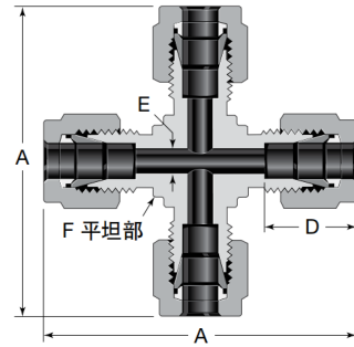
卡套四通 SKX
