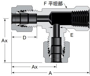
卡套变径内螺纹三通 SKTBNF
