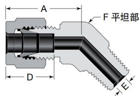
卡套45° 外螺纹弯通 SK4NM
