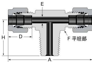
卡套变径外螺纹三通 SKTBNM
