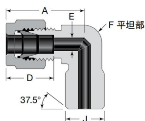
卡套90° 管外焊直角 SK9GW
