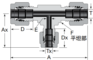
卡套变径三通 SKTB
