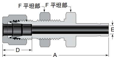
卡套穿板卡管直通 SKZCBKG
