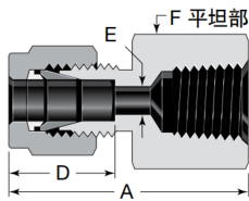
卡套内螺纹直通 SKZRC
