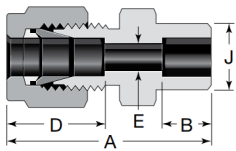
卡套承插焊直通 SKZCW
