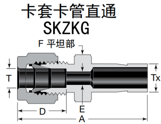
变径接头 (公制到英制)
