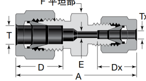
卡套变径直通 SKZB
