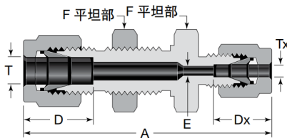
卡套穿板变径直通 SKZBCB
