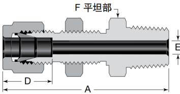
卡套穿板外螺纹直通 SKZCBNM
