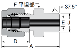
卡套管外焊直通 SKZGW
