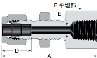
卡套穿板内螺纹直通 SKZCBNF
