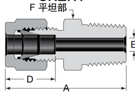
卡套外螺纹直通 SKZRT
