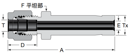
卡套长卡管直通 SKZCKG
