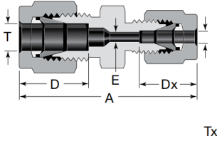
卡套变径直通 SKZB
