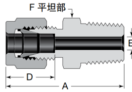
卡套外螺纹直通 SKZNM
