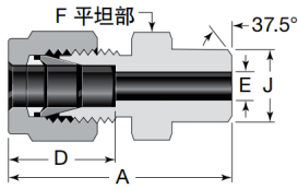
卡套管外焊直通 SKZGW
