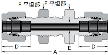
卡套穿板直通 SKZCB
