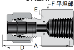
卡套内螺纹直通 SKZNF
