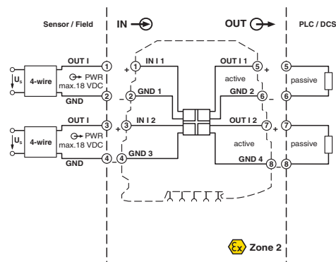
结构框图
