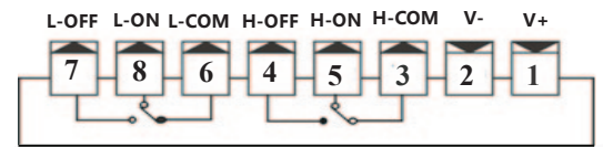
航插电缆定义图
