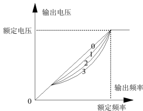
图 6-5 V/F 曲线
