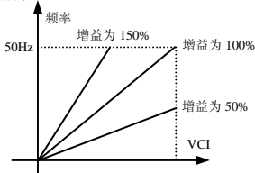
图 6-19: VCI 模拟输入增益
