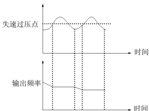
图 6-39 过压失速功能
