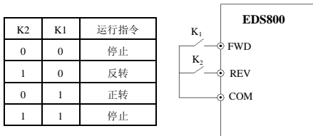
图 6-28 两线式运转模式 1
