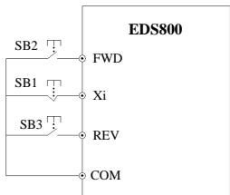
图 6-30 三线式运转模式 1
