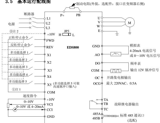
图 3-6 基本配线图
