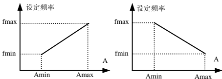
(1)正作用特性
