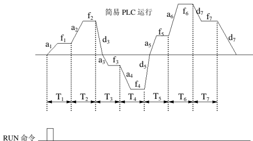
图 6-21 PLC 单循环后停机方式
