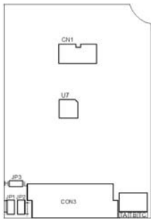
图 3-7 控制板的拨动开关位置示意图
