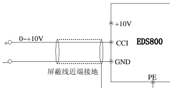
图 3-9 CCI 端子配线图
