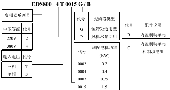
图 2-1 变频器型号说明
