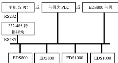
图 10-1 组网方式示意图
