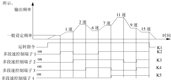
图 6-25 多段速运行示意图
