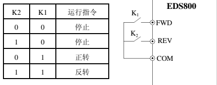
图 6-29 两线式运转模式 2
