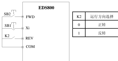
图 6-31 三线式运转模式 2
