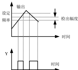
图 6-33 频率到达信号输出示意图
