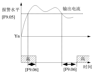
图 6-38 过载报警
