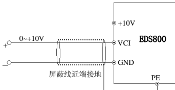
图 3-8 VCI 端子配线图
