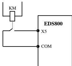
图 6-27 外部设备故障常开输入示意图
