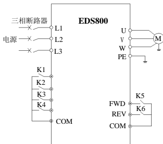
图 6-26 多段速运行接线图
