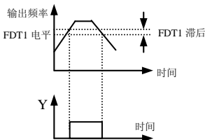
图 6-34 频率水平检测示意图
