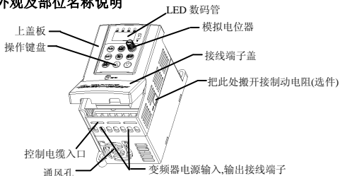
图 2-3 变频器各部位名称示意图
