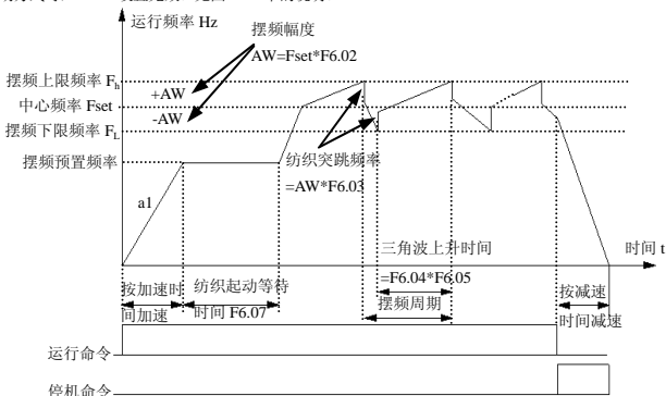
图 6-36 摆频示意图
