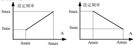
(2)反作用特性
