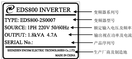
图 2-2 变频器铭牌
