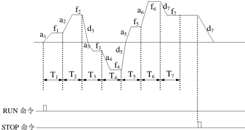
图 6-22 PLC 单循环后保持方式
