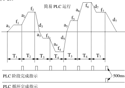
图 6-20 简易 PLC 运行图
