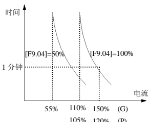
图 6-37 电子热继电器保护
