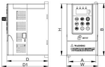
图 2-4 外形图
