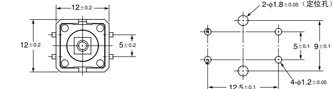
印刷基板孔加工尺寸条例 (TOP VIEW) (单面基板 t=1.6)
