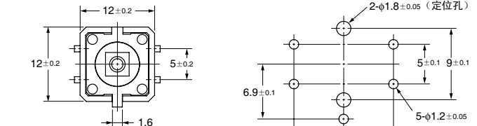
印刷基板孔加工尺寸条例 (TOP VIEW) (单面基板 t=1.6)
