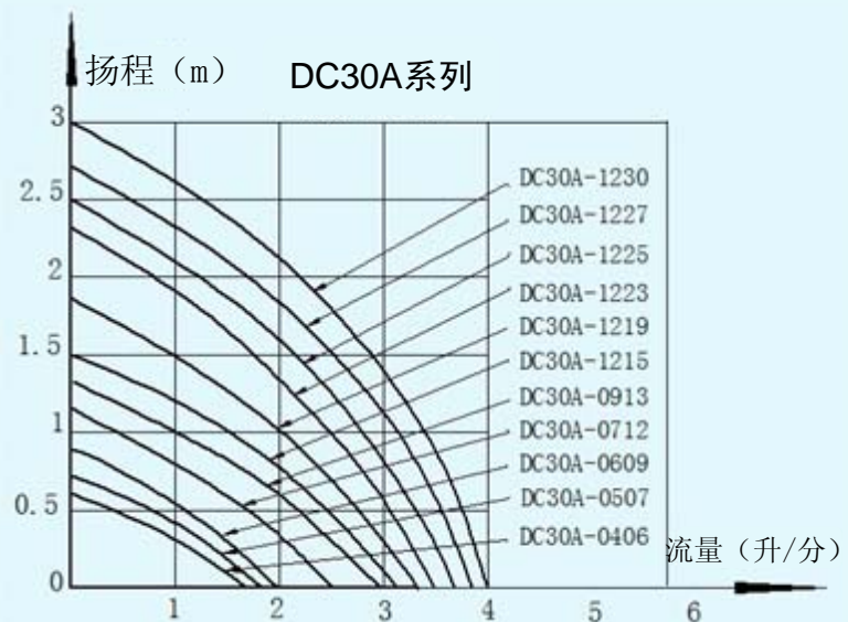
扬程-流量曲线图
