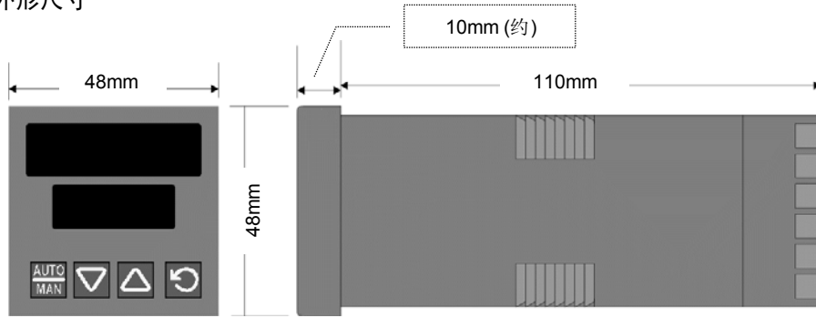
外形尺寸
