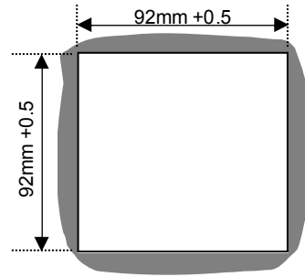
开孔尺寸
