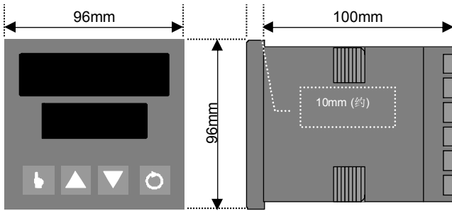
外形尺寸
