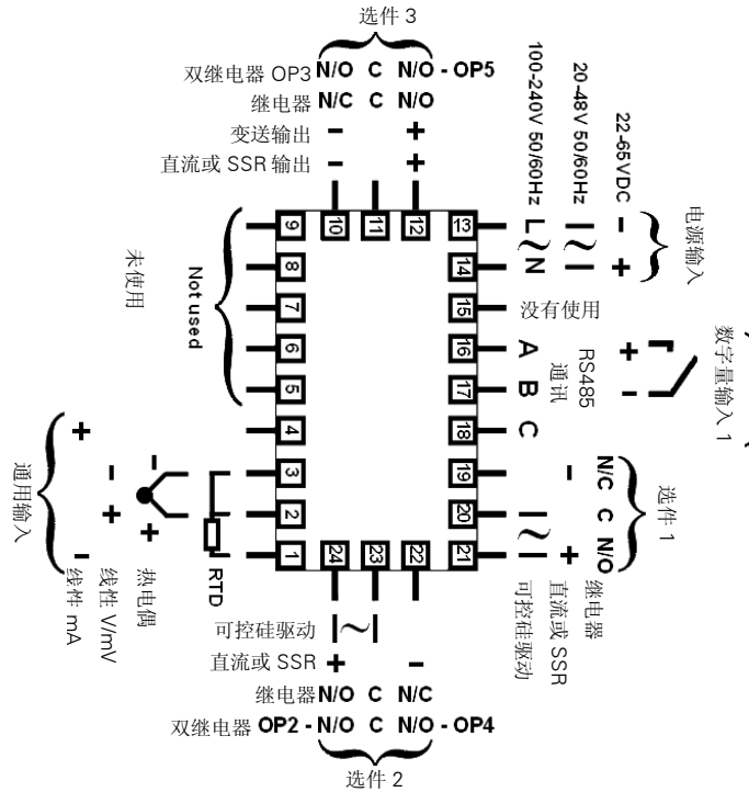
接线图
