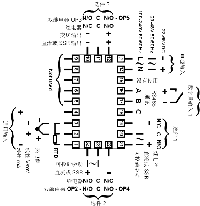
接线图
