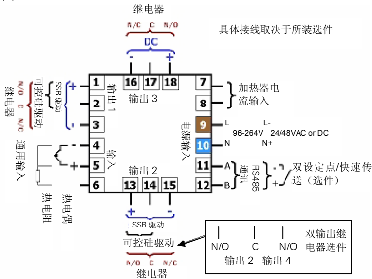
接线图
